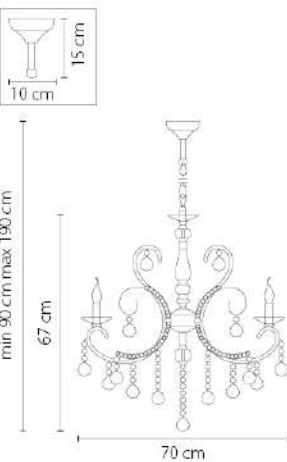
Схема с габаритными размерами:
